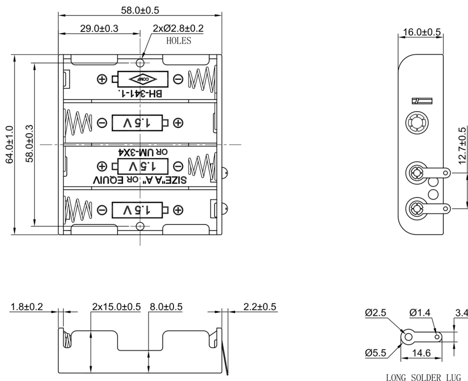
LONG SOLDER LUG
